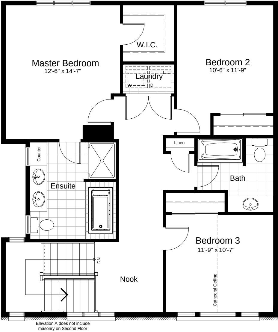
Elevation A, B & C
